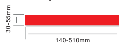
头卡尺寸图 Top card size
