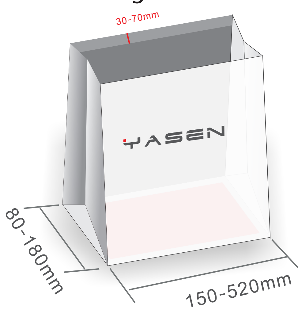
纸袋示意图 Bag size
